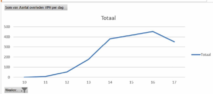
Figuren GHZ
